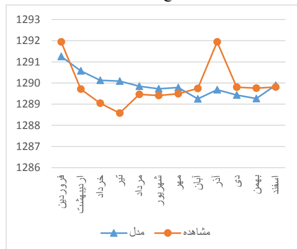
شکل ۷-۱۹ مقایسه نتایج مدل در چاه مشاهده ای اراضی حسین آباد
