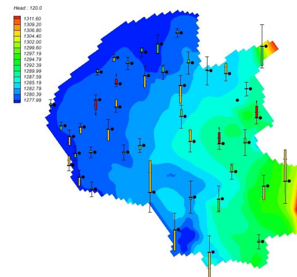
شکل ۳۰-۵ تراز آب محاسبه شده در خرداد ماه (بر حسب متر)
