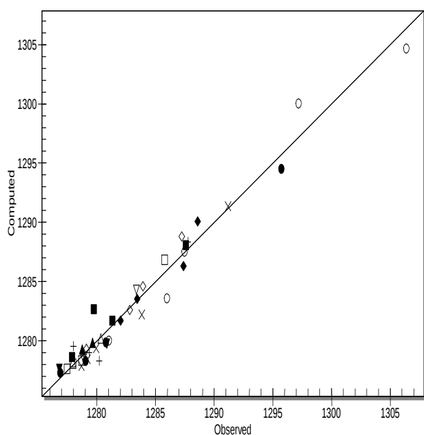
شکل ۴۹-۵ تفاوت مقدار محاسبه شده و مشاهده شده برای پیزومترها در تیر ماه (برحسب متر)
