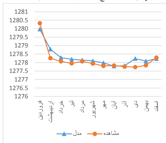
شکل ۷-۹ مقایسه نتایج مدل در چاه مشاهده ای فسدوزشیات
