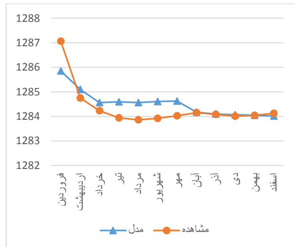
شکل ۷-۱۷ مقایسه نتایج مدل در چاه مشاهده ای بکتابش
