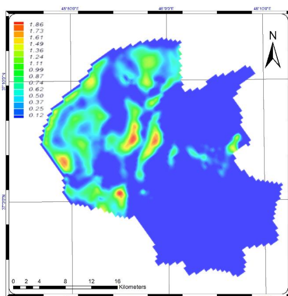
شکل ۴۲-۵ نقشه توزیع تبخیر صورت گرفته از آبخوان در سطح دشت (برحسب میلی متر در روز)
