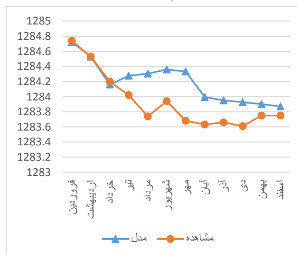
شکل ۷-۶۰ مقایسه نتایج صحت سنجی در چاه مشاهده ای ابکناش
